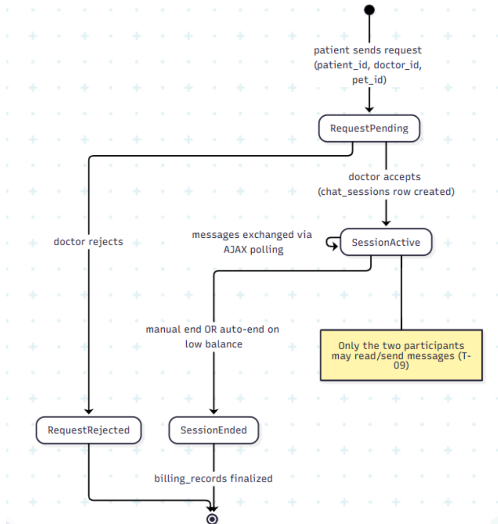
Fig-1: Chat Session
